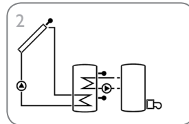
Zonnestelsysteem met naverwarming (pagina 11)
