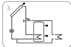
Standaardzonnestelsysteem met restwarmteafvoer (pagina 16)
