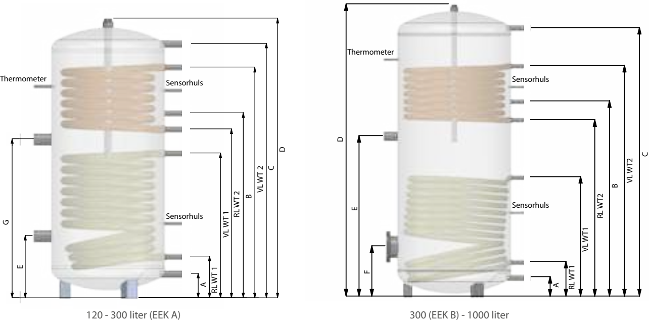
Schematische weergave
