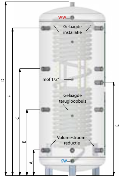
Schematische weergave
