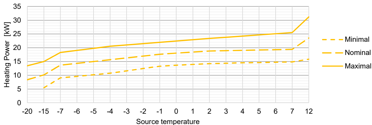
Heating Power WPLT829 bei Vorlauftemperatur 35°C*
