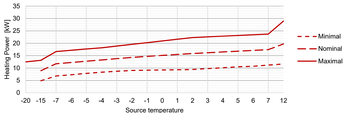
Heating Power WPLT829 bei Vorlauftemperatur 55°C*
