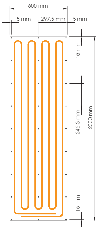
MWH F206 Verwarmingsoppervlak 1,2 m 2
