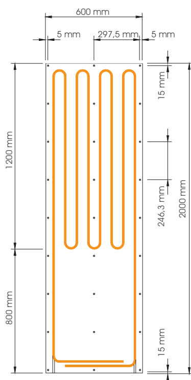
F206V Verwarmingsoppervlak 0,75 m 2
