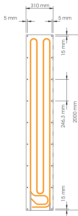
F 203 Verwarmingsoppervlak 0,625 m 2
