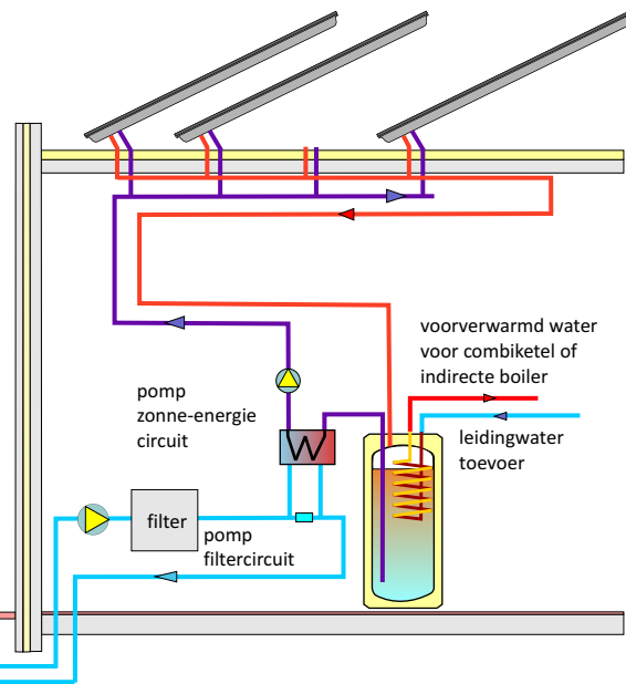
Figuur 1 Schematisch overzicht van de toepassing van een zonneboilersysteem bij buitenzwembaden.
